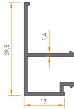
1993 KANAT TEK CAM ÇİTASI 0.330 kg/mt
