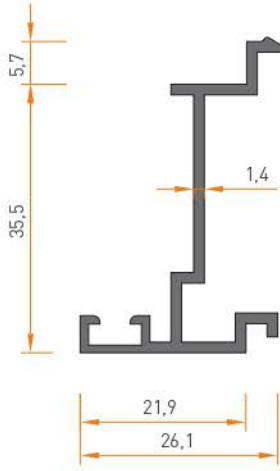
2019 KAPI KANAT ADAPTÖR 0.355 kg/mt
