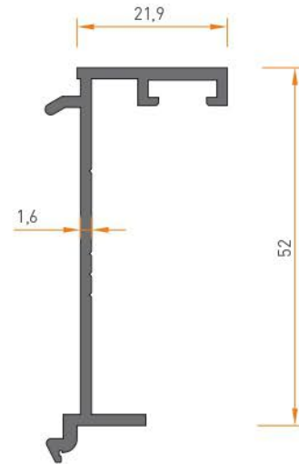
1987 KANAT ADAPTÖR 0.465 kg/mt
