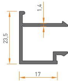
1986 KANAT ISI CAM ÇİTASI 0.270 kg/mt
