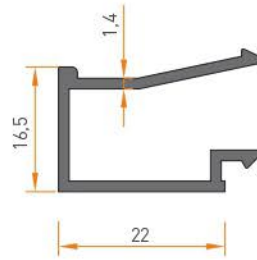
1985 KASA ISI CAM ÇİTASI 0.285 kg/mt
