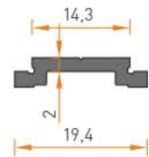
2641 SİSTEM TİJ 0.130 kg/mt
