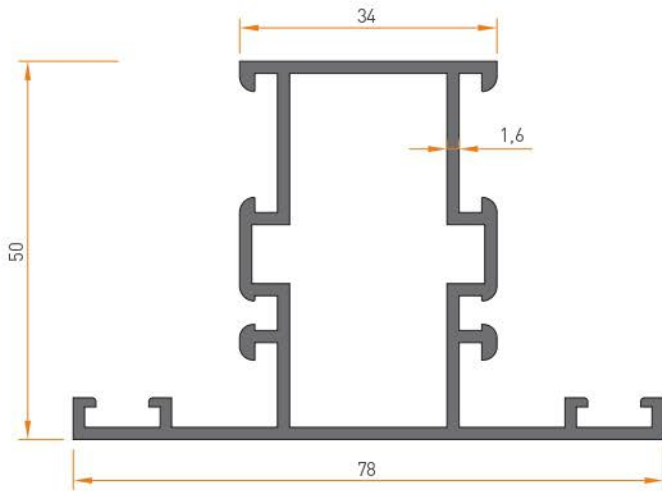
1991 ORTA KAYIT 1.175 kg/mt
