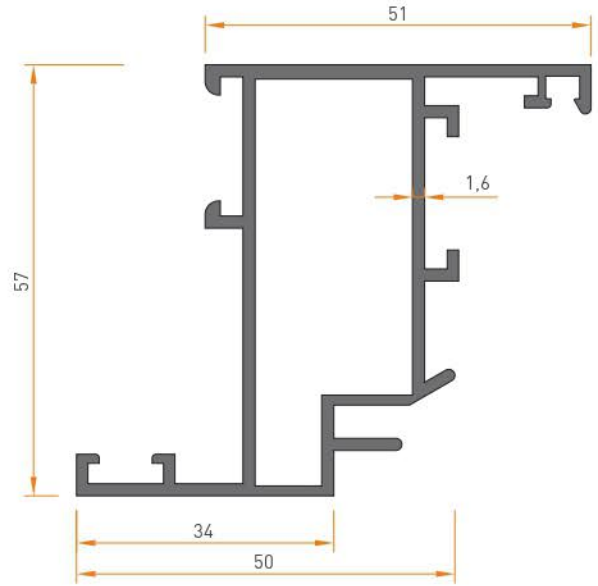
1992 KANAT 1.125 kg/mt
