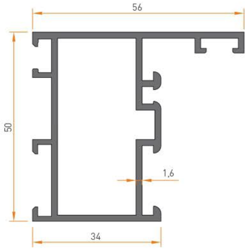
1994 KASA 1.000 kg/mt
