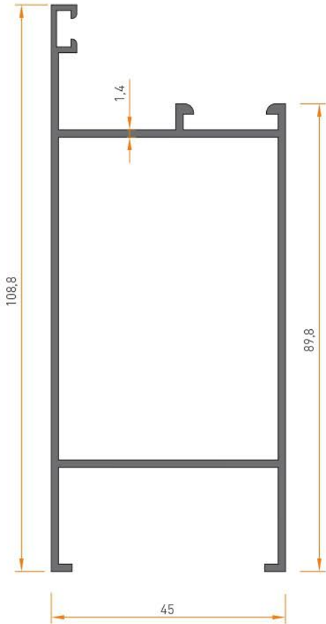
2010 ETEK PROFİL 1.150 kg/mt
