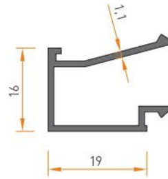
2012 ISI CAM ÇİTASI 0.205 kg/mt
