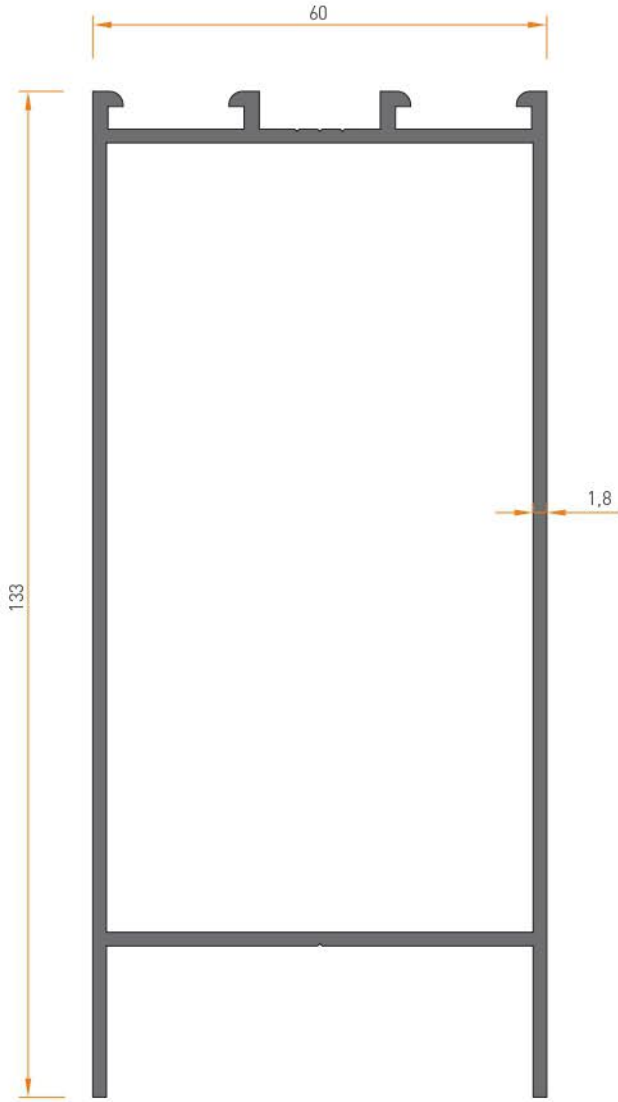
1982 ETEK PROFİL 1.945 kg/mt
