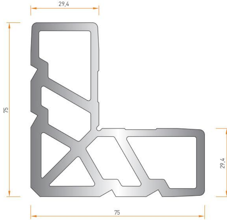
2533 KÖŞE TAKOZU 4.280 kg/mt
