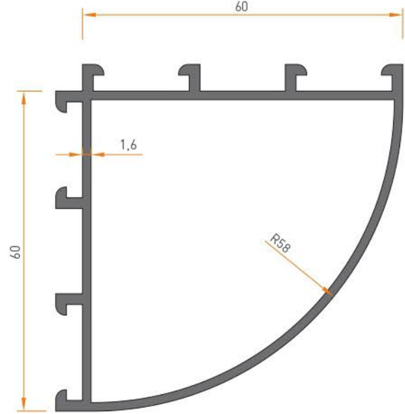
1983 KÖŞE PROFİL 1.195 kg/mt
