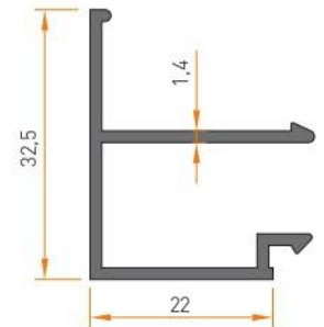
1995 KASA TEK CAM ÇİTASI 0.345 kg/mt
