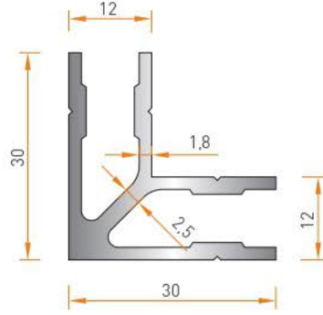
2142 KÖŞE TAKOZU 0.620 kg/mt
