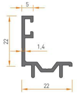
1990 TIRNAK 0.250 kg/mt
