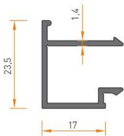
1986 KANAT ISI CAM ÇİTASI 0.270 kg/mt
