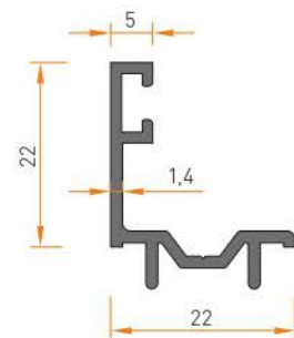
1990 TIRNAK 0.250 kg/mt
