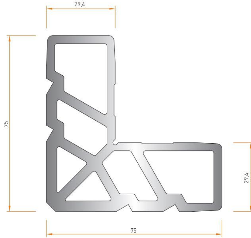
2533 KÖŞE TAKOZU 4.280 kg/mt
