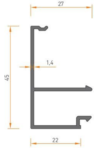
1974 ÇİTA 0.410 kg/mt
