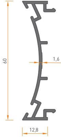
1989 ÇARPMA KAPI ADAPTÖR 0.460 kg/mt
